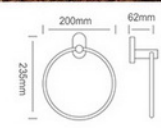
KD-3810 毛巾环 / Towel ring 材质: SUS 304 工艺: 亮光 箱容: 40
