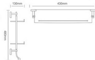
KD-3903B-2 二层置物架 Double layer glass shelf 材质: SUS 304 工艺: 亮光 箱容: 10
