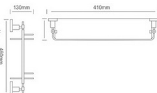
KD-3803-2 二层置物架 Double layer glass shelf 材质: SUS 304 工艺: 亮光 箱容: 10
